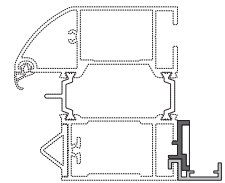
Profilé complémentaire de recouvrement du doublage
