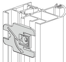
Bride pour Thermo46 Exemple sur huissérie A1
