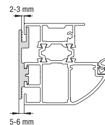
Huissérie en aluminium A1 avec bride de fixation pour Thermo46
