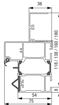
Huisserie A4 avec tapée
