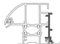
Profil complémentaire de recouvrement du doublage
