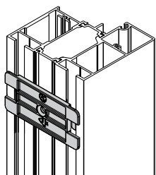
Bride pour Thermo65 Exemple sur huissérie A1
