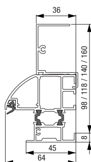
Huissérie A1 avec tapée
