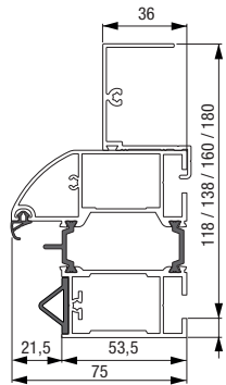
Huisserie A3 avec tapée
