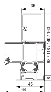
Huissérie A2 avec tapée
