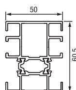
Profilé d'élargissement 50 mm
