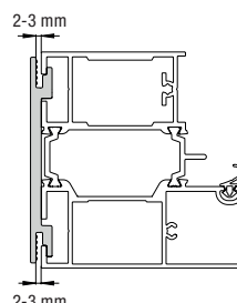
Huissérie en aluminium A4 avec bride de fixation pour Thermo65
