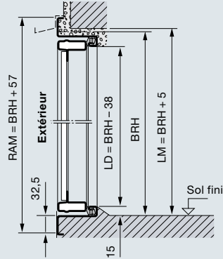
A 1 vantail avec seuil
