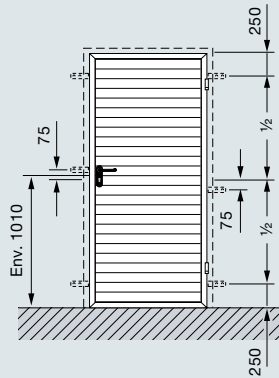
A 1 vantail sans seuil
